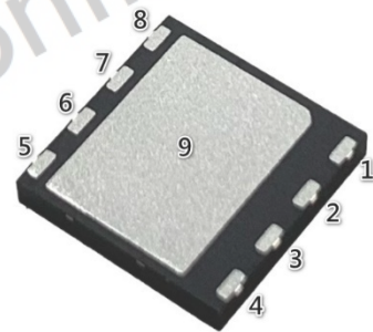
INF-065C120AGA: (PDFN8 8x8 mm)
