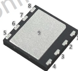
INF-065D090AGA: (PDFN8 8x8 mm)
